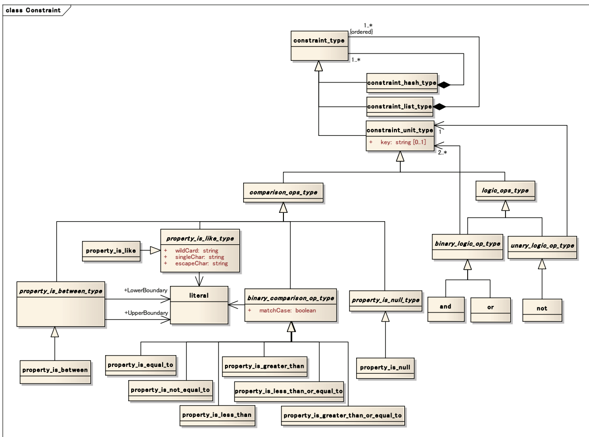
Figure 4 RTC プロファイル(制約部分)
