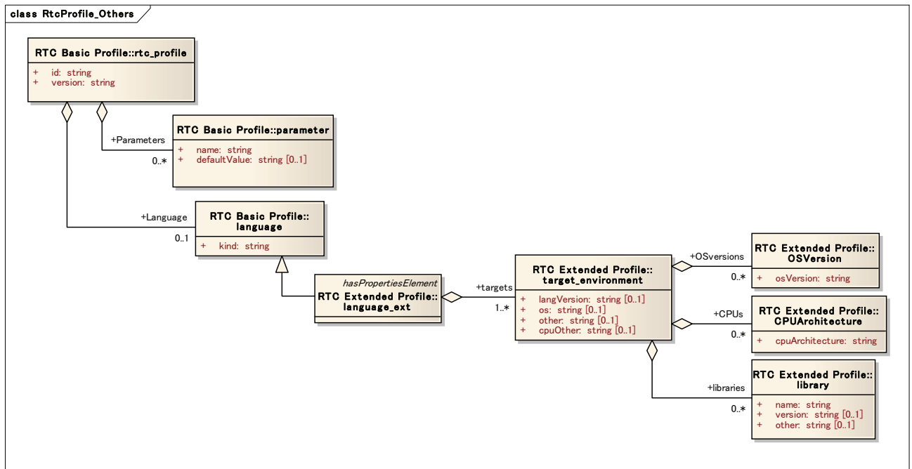
Figure10 RTC プロファイル(パラメータ, 言語部分)
