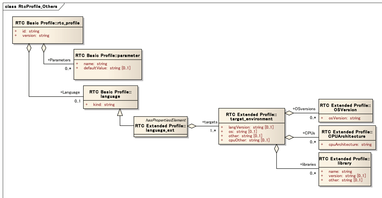
Figure 21 RTC プロファイル(言語部分)
