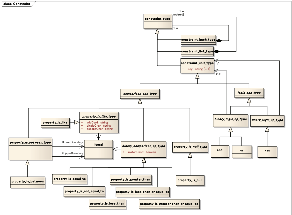
Figure 11 RTC プロファイル(制約部分)
