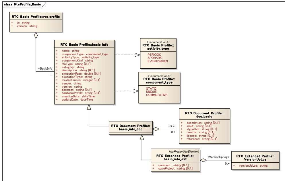
Figure 12 RTC プロファイル(コンポーネント部分)
