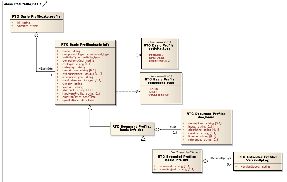
Figure 5 RTC プロファイル(コンポーネント部分)
