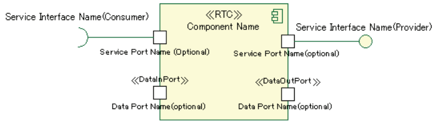
図 1 RT コンポーネント構成図凡例 (RT コンポーネント単体)
