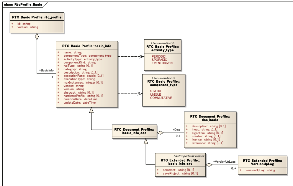
Figure17 RTC プロファイル(基本部分)
