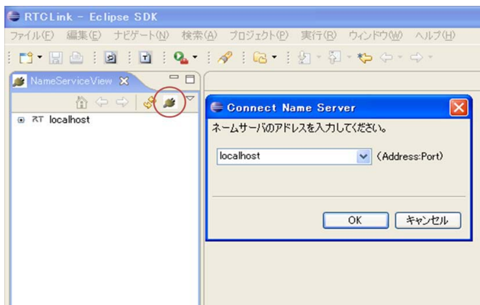
図 2 Eclipse の画面
