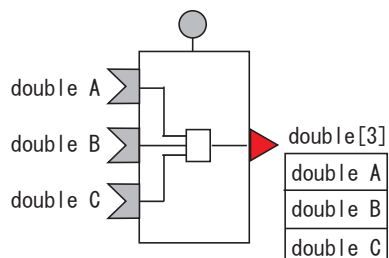
図3 Multiplexer コンポーネント
